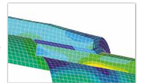
Analiza napetosti zlepljenih cevi
