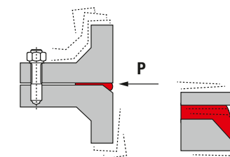
Slika 3: lepilo & tesnilo
