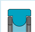
Profil TCS 120
